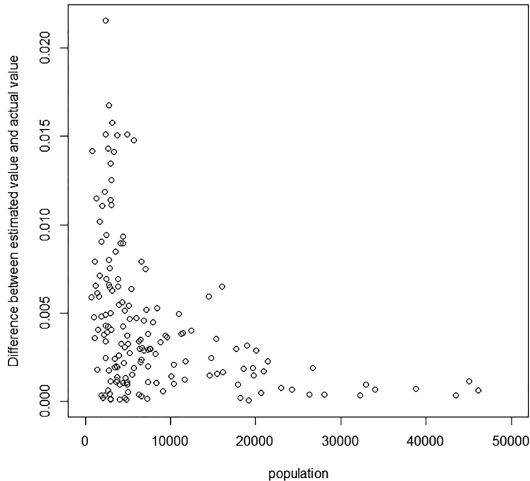
図 8 出生率指数と単純出生率の差と人口との関係
