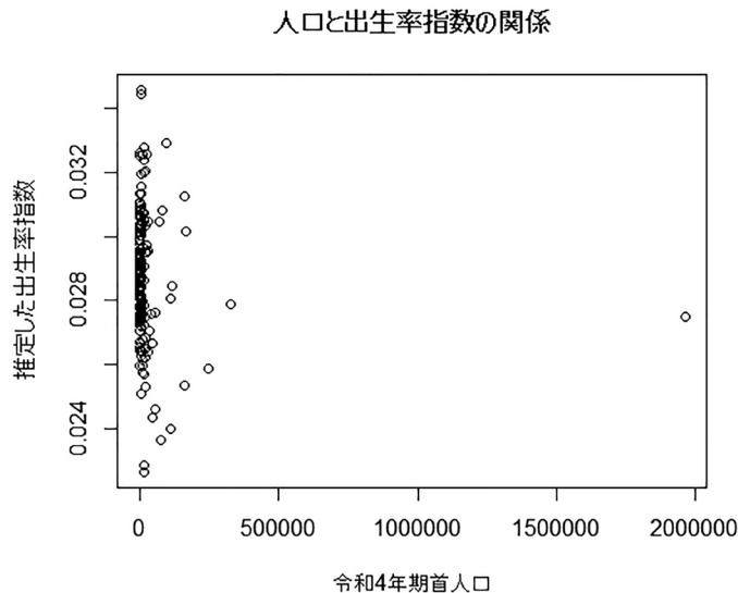
図6 人口と出生率指数との関係
