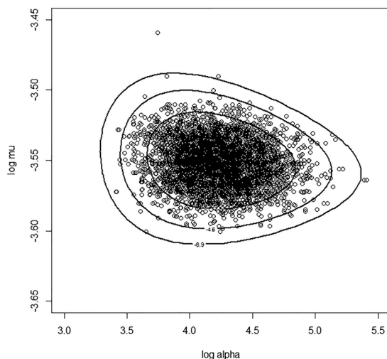
図 4 推定した超パラメーターの対数値の分布
