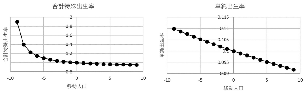
図 2 移動人口と合計特殊出生率及び単純出生率の関係
