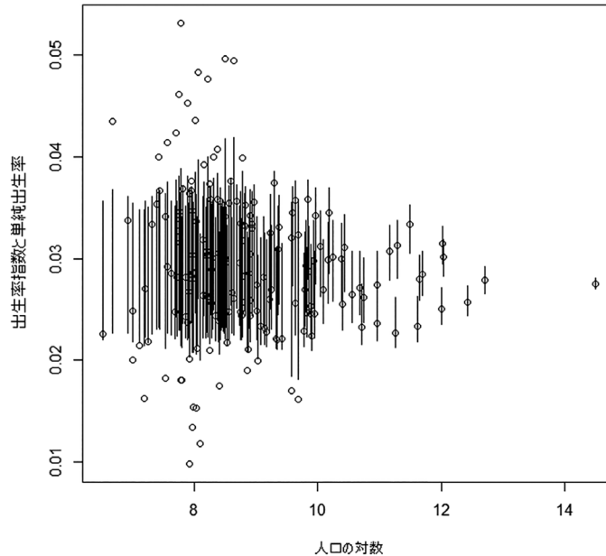
図7 人口と出生率指数及び単純出生率の関係 (縦棒は自治体毎の出生率指数 95% 信頼区間を示す)
